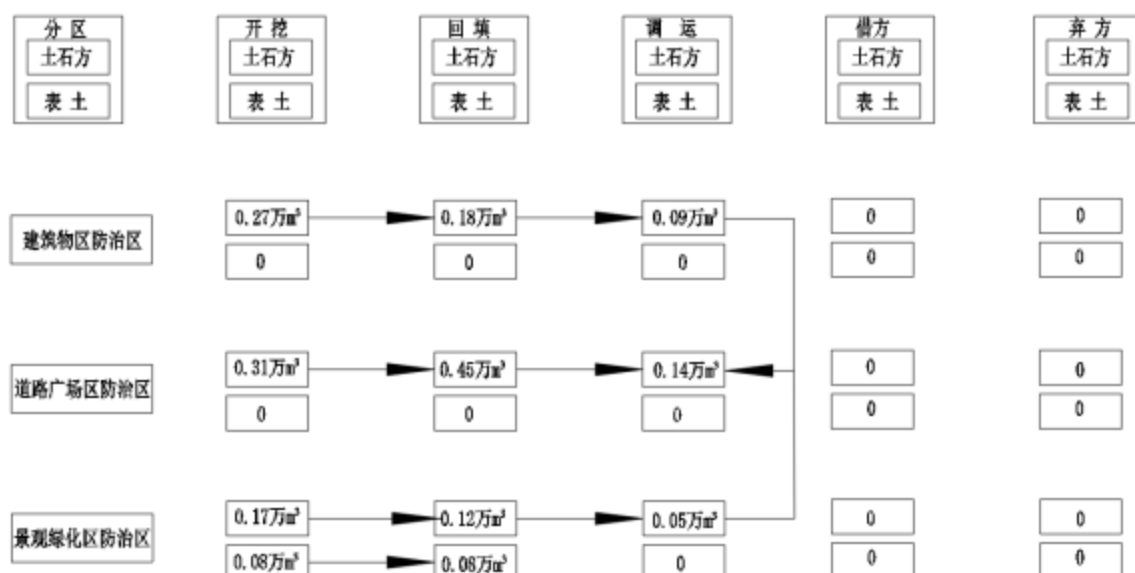
图 1-3 土石方流向框图
